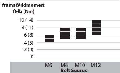
Joonis A— Käega lünni keeratud
