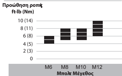
Εικόνα Α — Σφίξιμο με το χέρι
