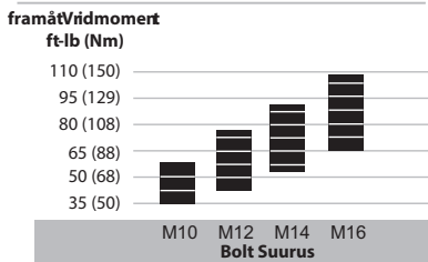
Joonis B— Vötmega lünni keeratud
