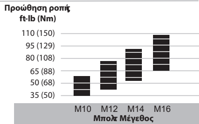
Εικόνα Β — Σφίξιμο με κλειδί
